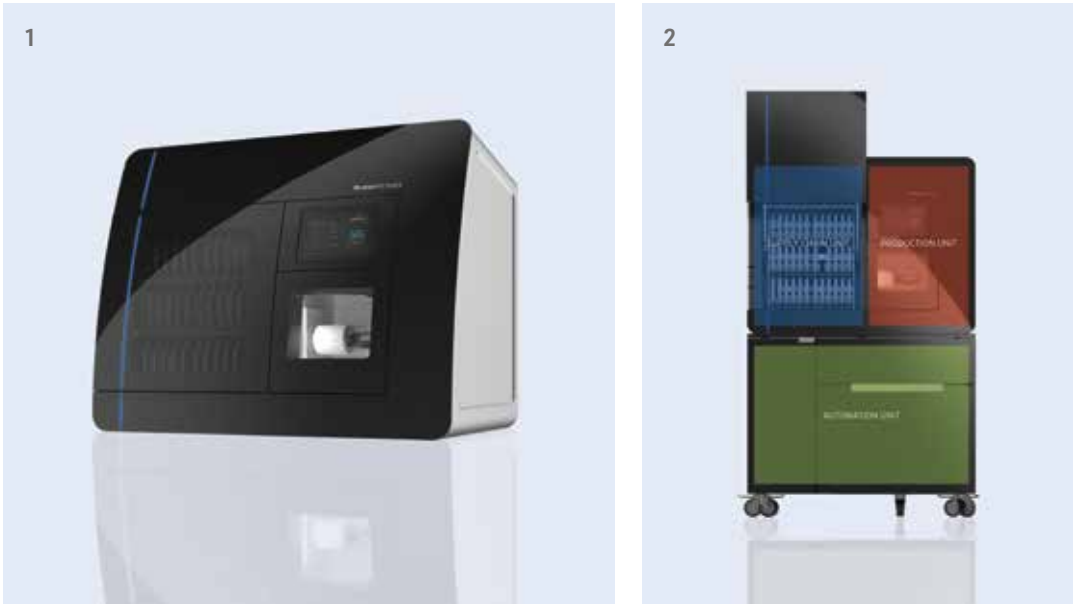
Fig. 1: Ceramill Matik; Fig. 2: Ceramill Matik unisce tre apparecchi in uno: la stazione di lavorazione vera e propria, un sistema totalmente automatico di gestione del magazzino e una unità di pulizia integrata.
